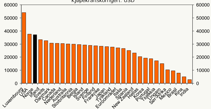
BNP pr. innbygger. 2003 Kjøpekraftskorrigert. USD
